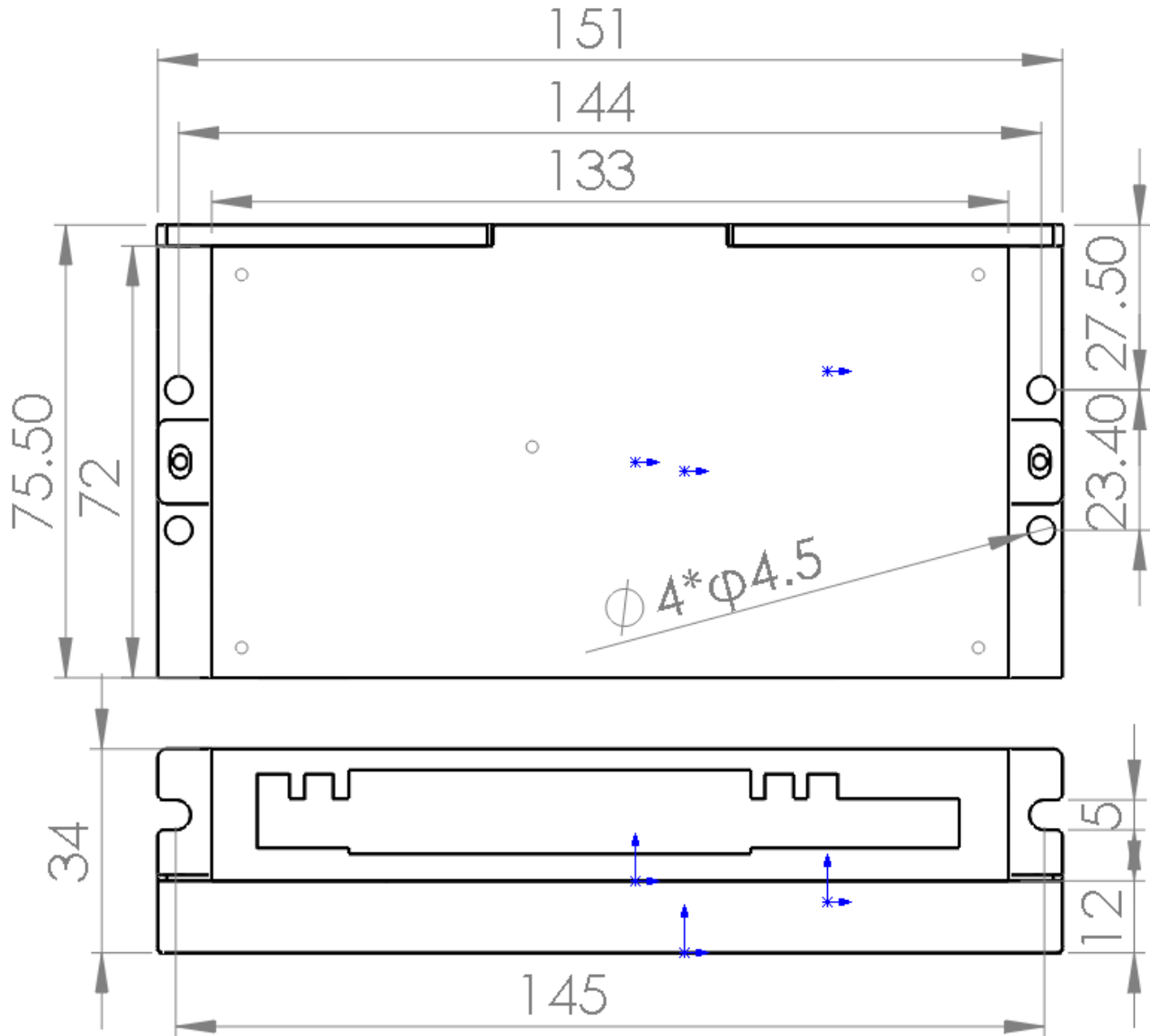
图 3.1-1 L2DB 伺服驱动器安装尺寸
