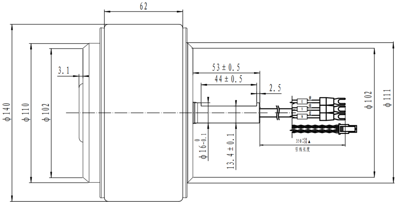
图 3.1-6 5.5 寸 15Nm 轮毂电机安装尺寸
