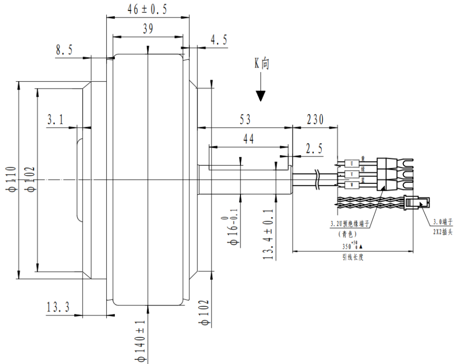
图 3.1.2 5.5 寸轮毂电机安装尺寸
