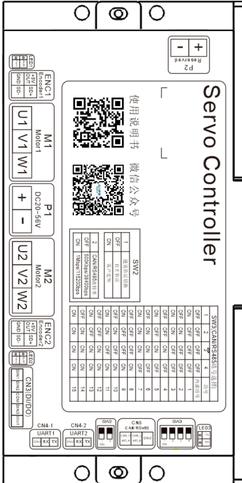
4.1.1 外壳丝印
